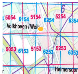
Abb. 4.6: Anordnung der Gitternetze (blau: Gauß-Krüger-System, rot: ETRS89/UTM)
