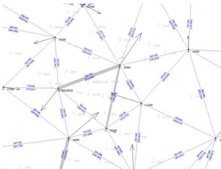
Abb. 3.1: Darstellung eines Sysplans zu einer Diagnoseausgleichung
