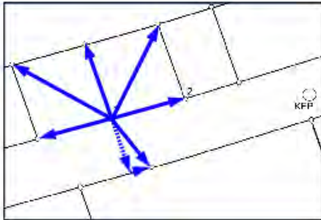
Abb. 2.13: Koordinatendifferenzen sind Beobachtungen für die Ausgleichung
